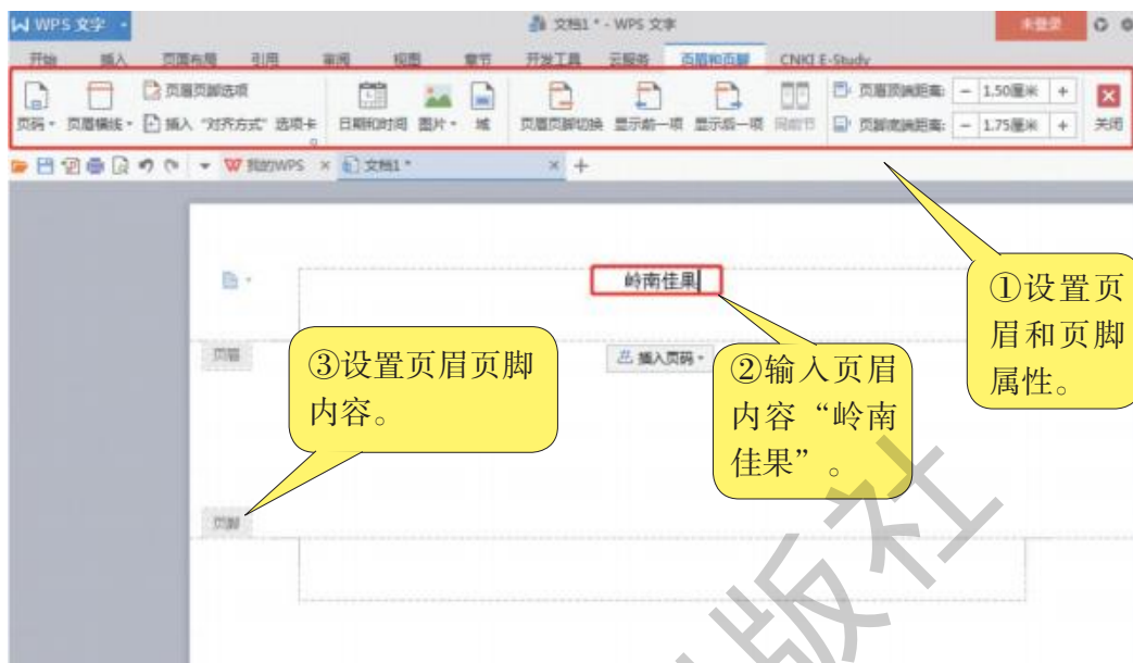
图3-5 编辑页眉和页脚
