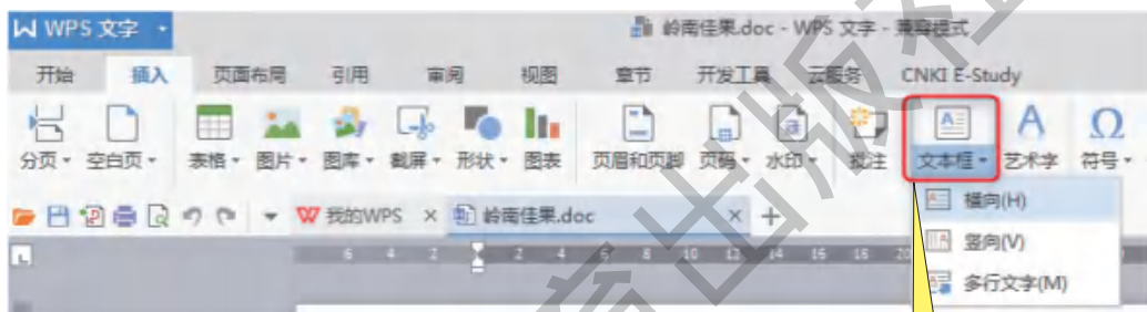
图3-11 插入文本框
