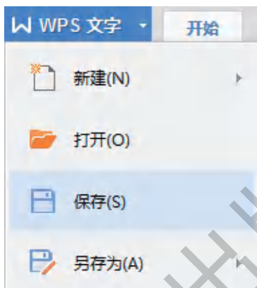
图2-3 保存文档
