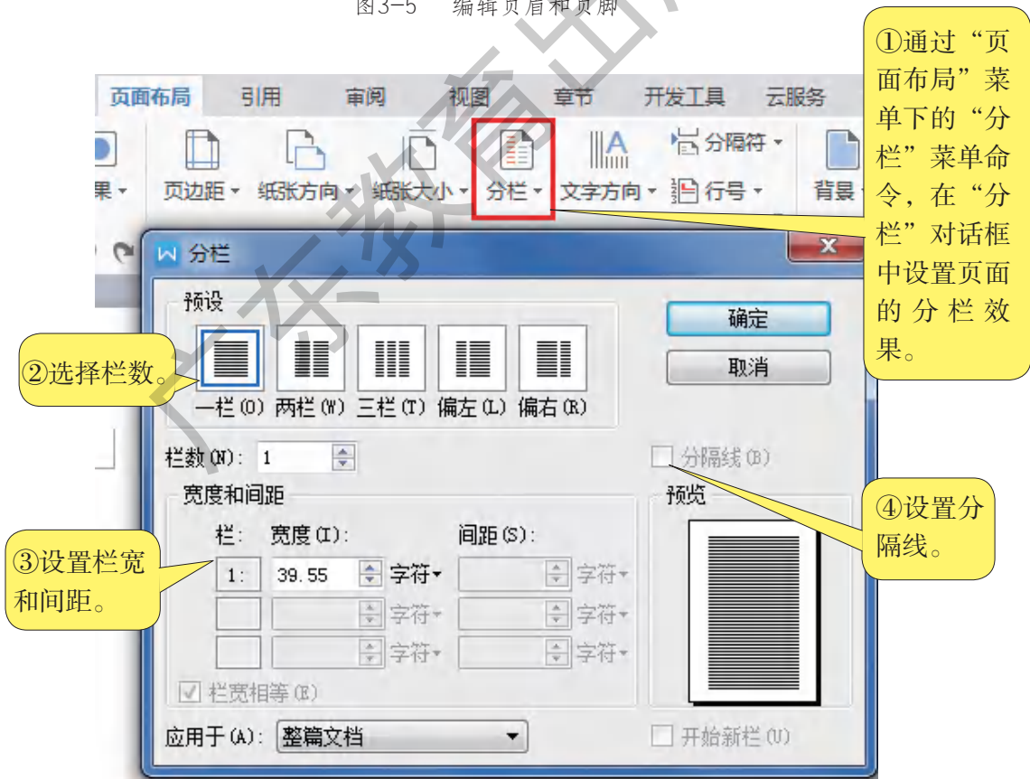
图3-6 设置分栏
