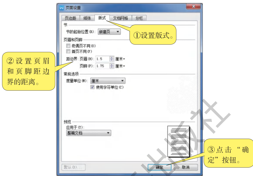
图3-3 设置版式
