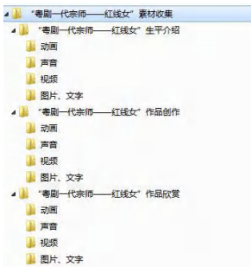
图9-1 分类文件夹
