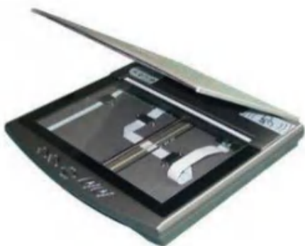
图9-2 扫描仪
