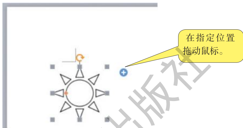
图5-2 绘图示范
